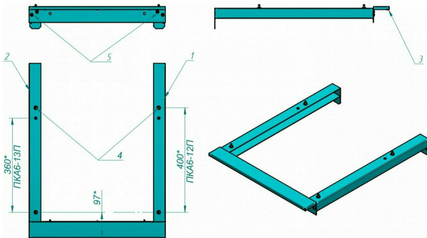
Схема сборки КСП6-12П и КСП6-13П
