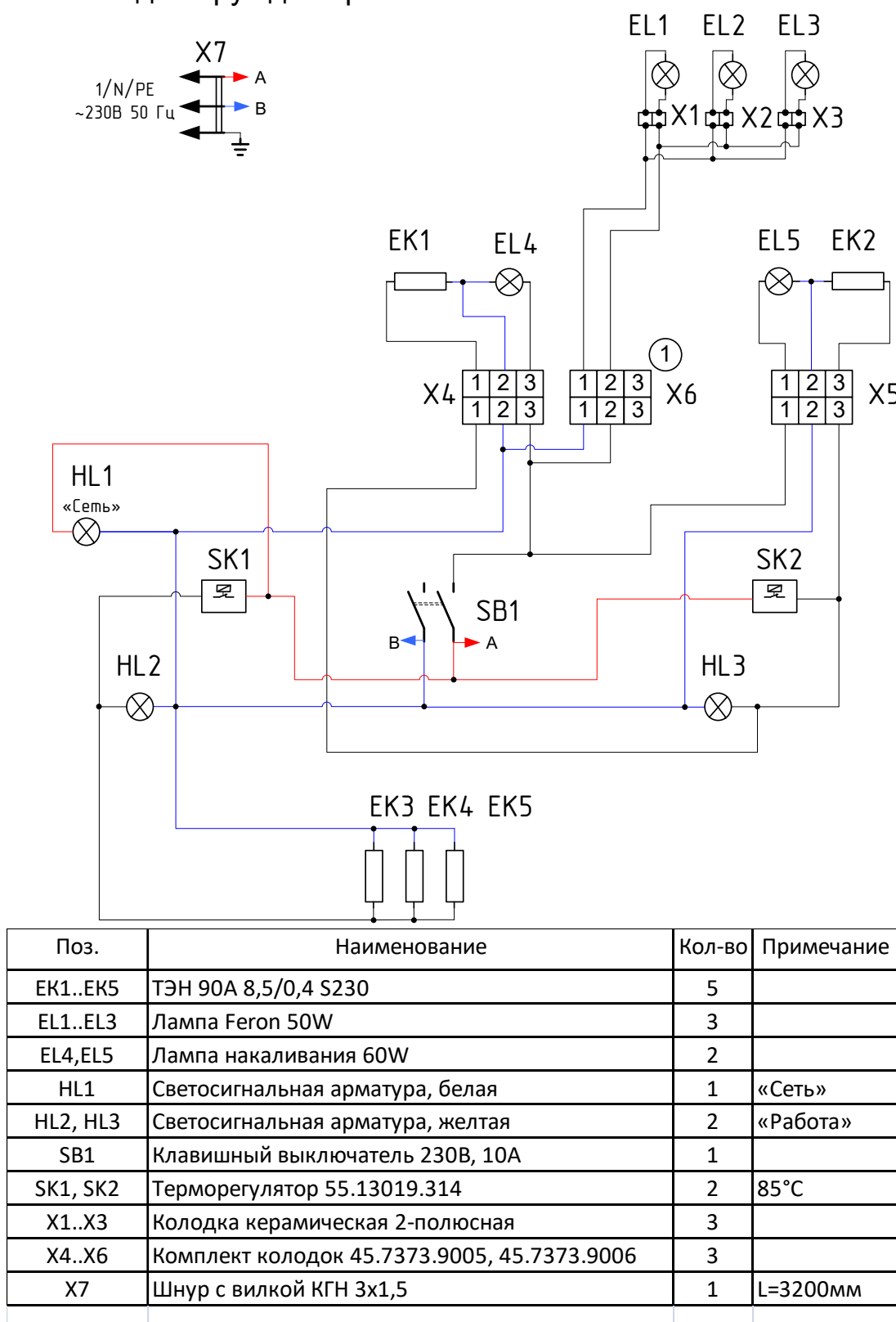
Рис.2 Схема электрическая принципиальная ВТН70
