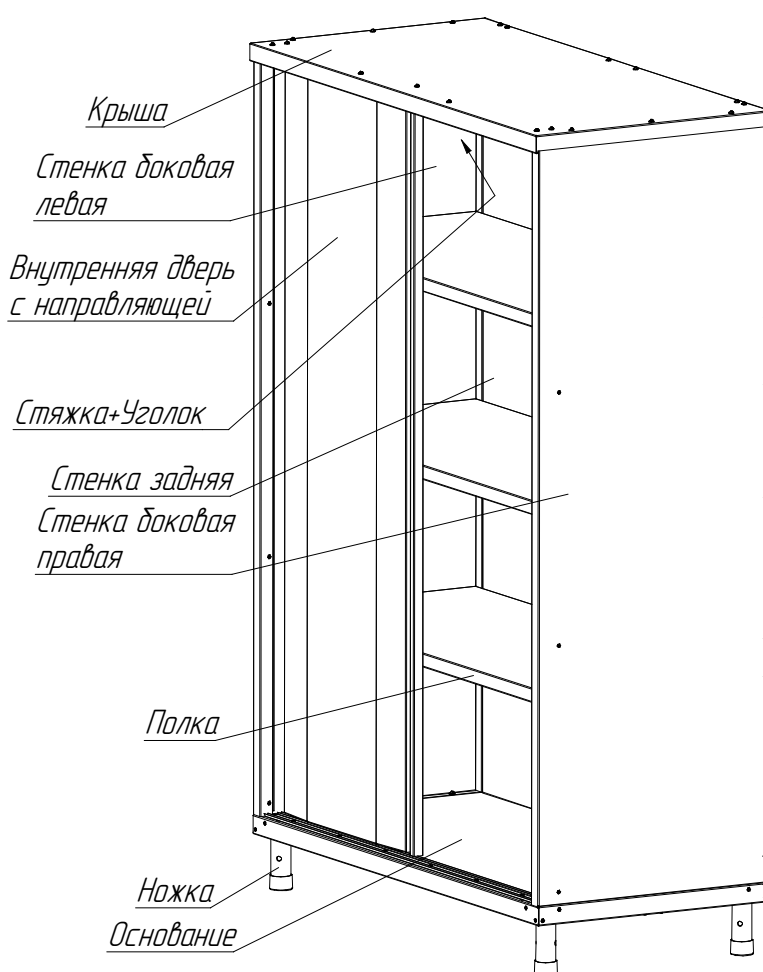
Рис.1 Внешний вид (Наружная дверь условно не показана)
