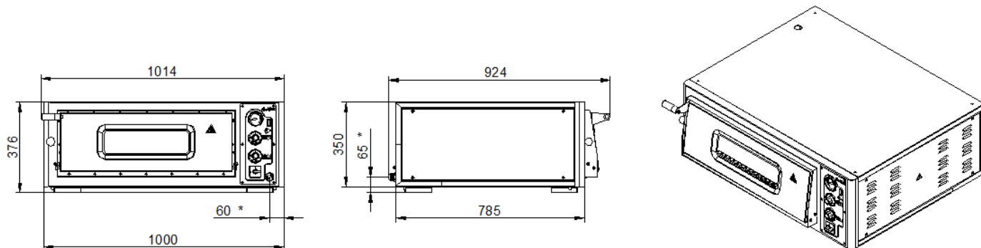
Рис. 1 - Общий вид печи ПЭП-4
